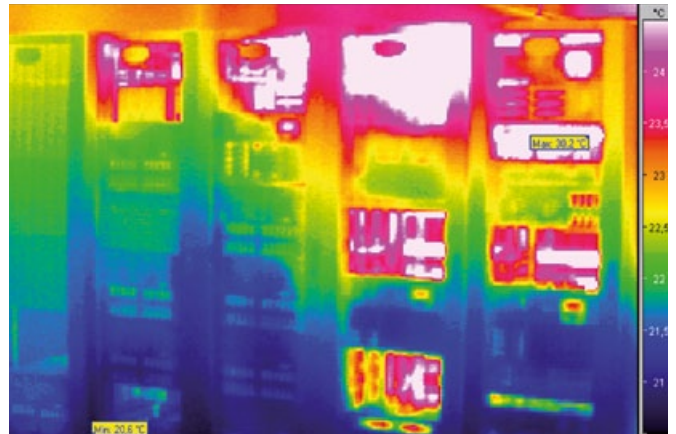
Una imagen termográfica visualiza las zonas calientes y frías del centro de datos, como sucede en un mapa meteorológico. Ello le permite detectar situaciones críticas en el sistema de aire acondicionado que provocan un aumento del consumo.
